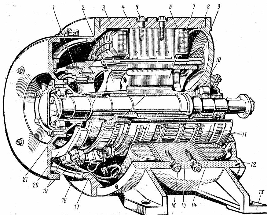
Рисунок 1 – Электродвигатель НБ-431
