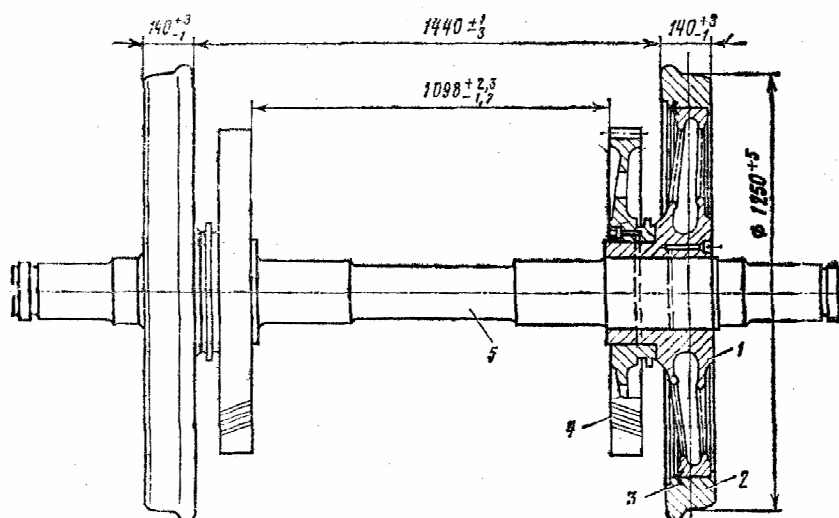
Рис. 1. Колесная пара электровоза
