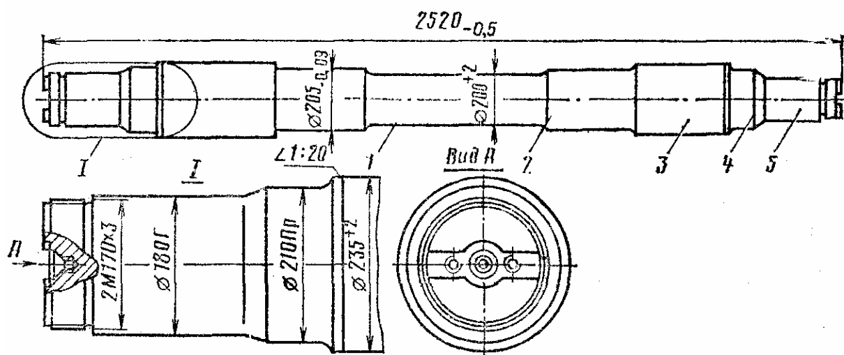
Рис. 2 Ось
