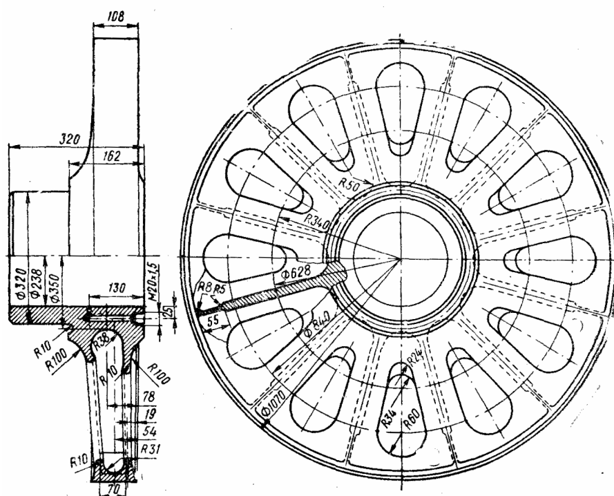
Рис.3 Колесный центр
