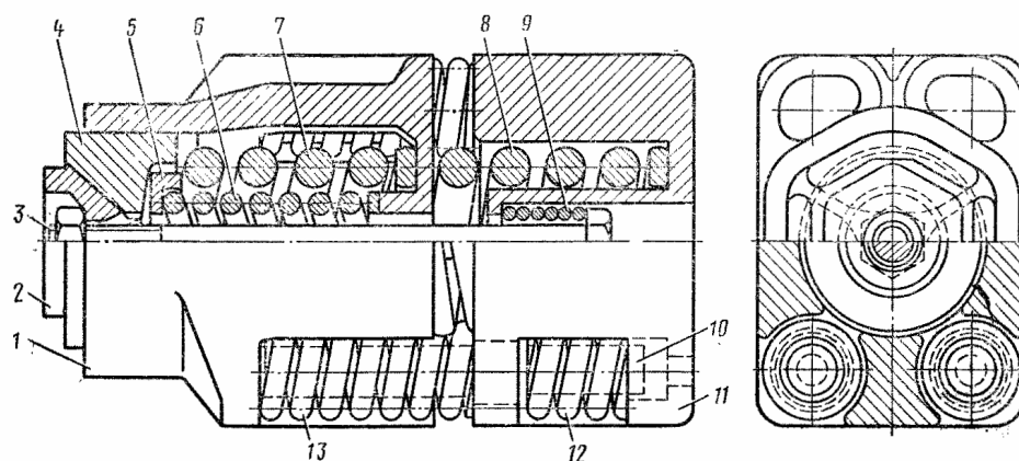
Рисунок 5 – Поглощающий аппарат ЦНИИ-Н6
