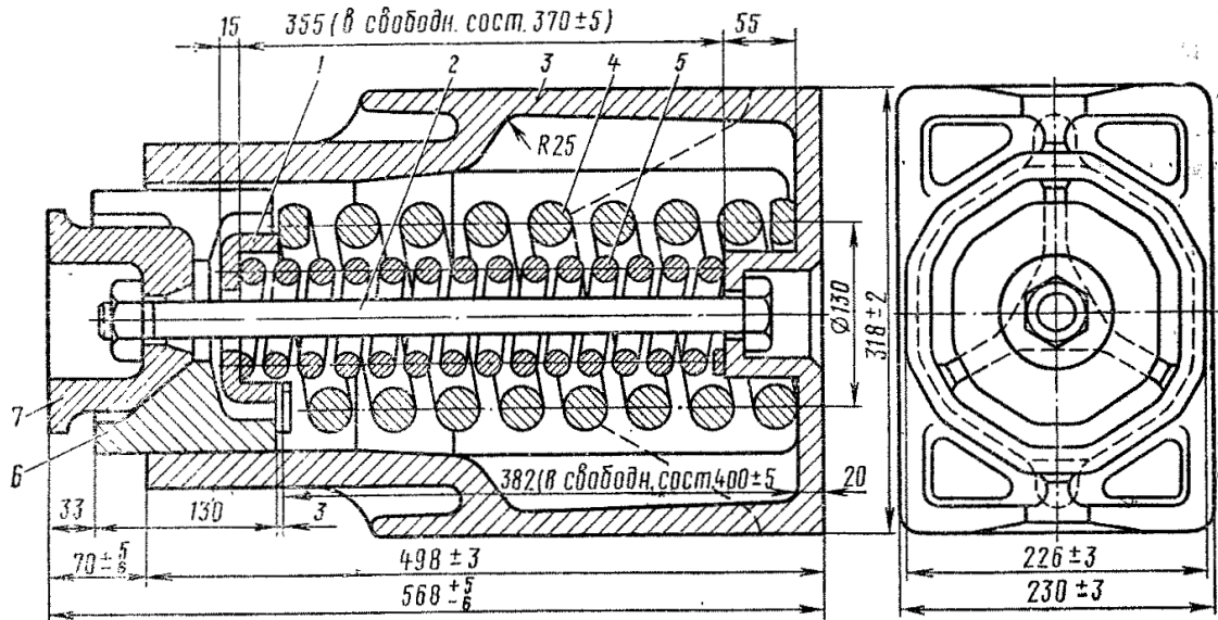
Рисунок 4 – Шестигранный поглощающий аппарат
